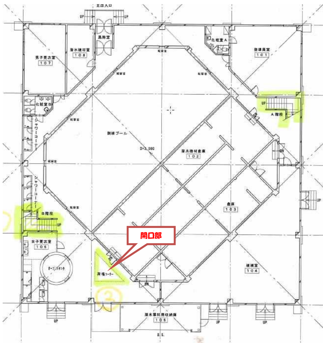
プール棟 1 階の平面図
